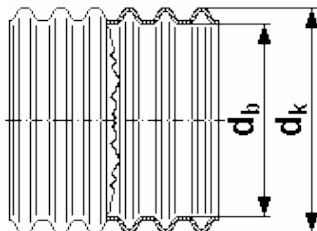
1. ábra - dréncső
